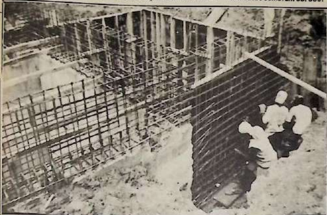
A estrutura de concreto da elevatória de Groenlândia.
